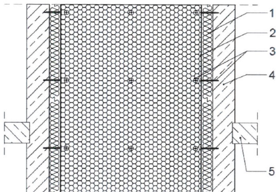
Przekrój A-A
