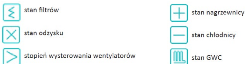
Rys. nr 37 Ikony statusu elementów układu zadajnika ADVANCE
